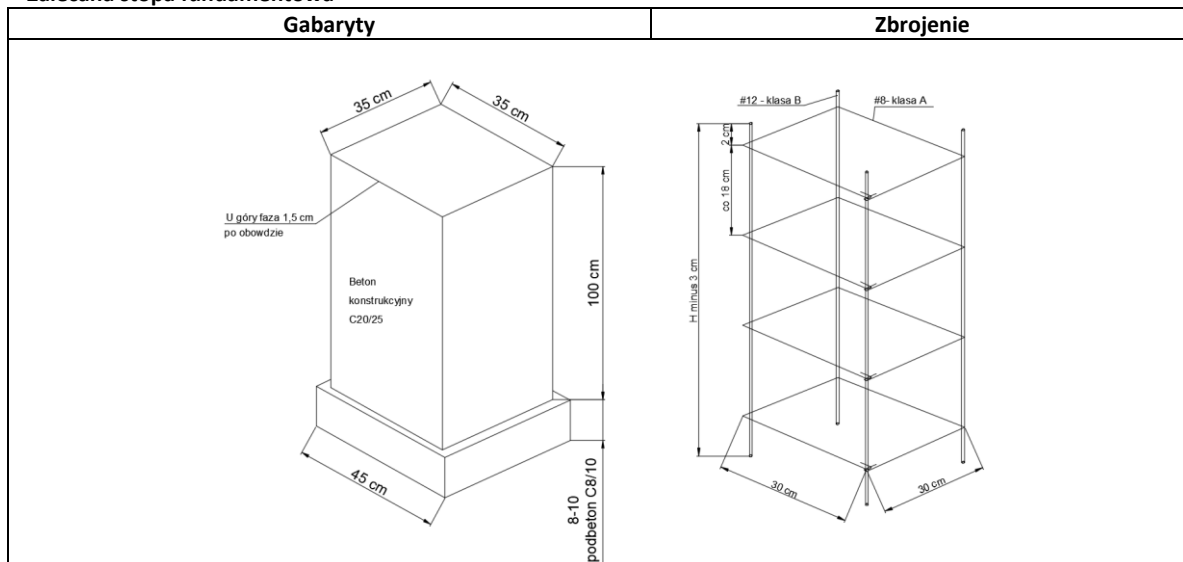
Rys. 34 Kształt i zbrojenie stopy fundamentowej
